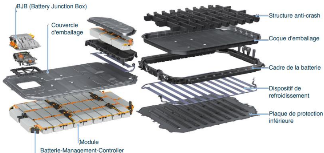
Figure 3: Structure d'une batterie dans son ensemble (RWTH Aachen, 2022b).
