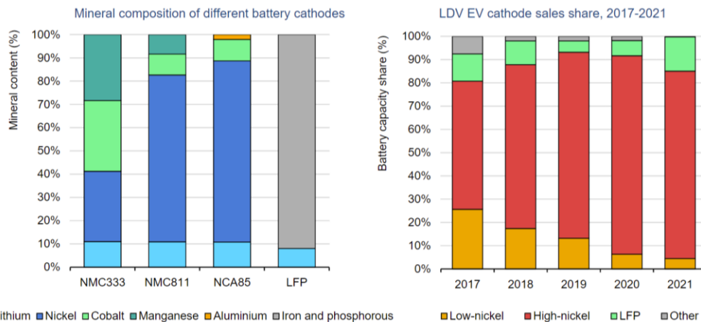
Figure 6: Composition en matériaux de différents types de cathodes (à gauche) et contribution de chaque type à la capacité globale des batteries (à droite) jusqu'en 2021 (AIE, 2022). LDV : light-duty vehicle (voitures particulières et véhicules utilitaires légers).
