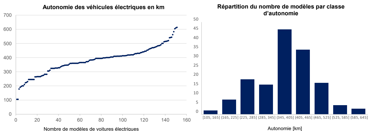
Figure 23: Aperçu de l'autonomie de tous les modèles de véhicules électriques disponibles sur le marché suisse. Graphique INFRAS sur la base des données d'Eco-Auto (2022).
