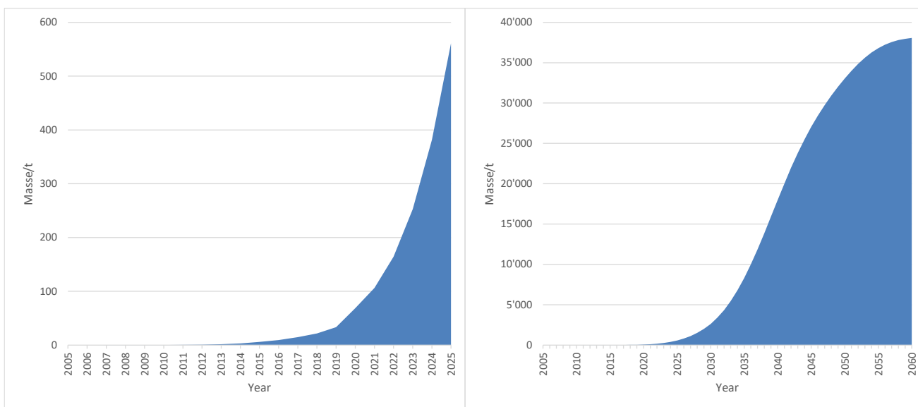
Figure 38: Projctions des flux de recyclage des batteries lithium-ion de véhicules électriques en Suisse d'ici 2025 (à gauche) et 2060 (à droite) (Widmer et al., 2021).
