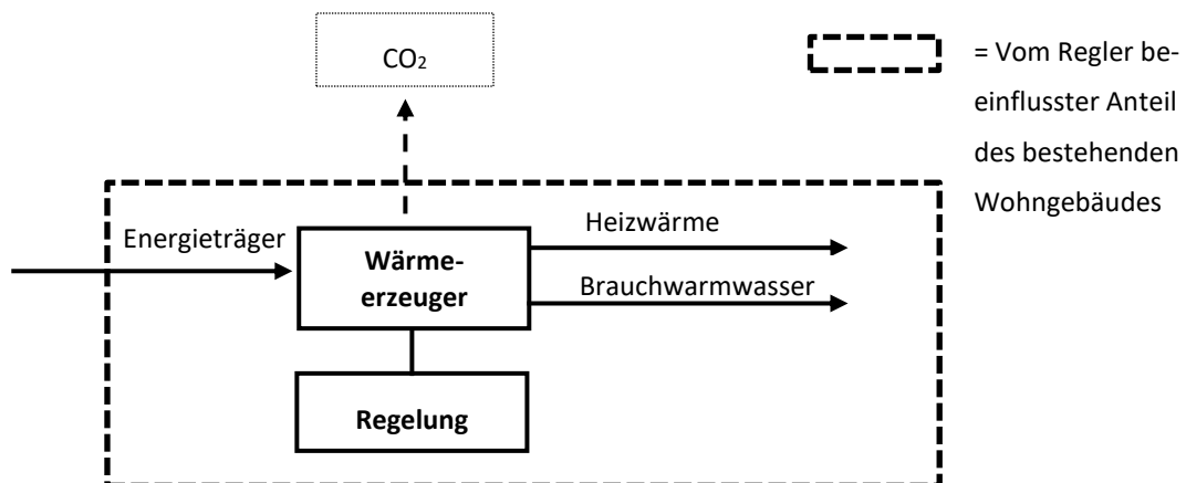
Abbildung 1: Schematische Darstellung der Systemgrenzen eines Vorhabens der Standardmethode
