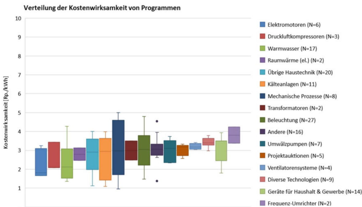
Abbildung 21: Verteilung der Kostenwirksamkeit von Programmen nach technischer Ausrichtung
