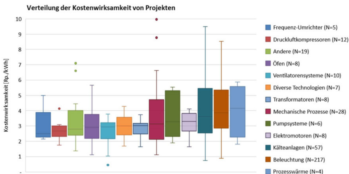
Abbildung 20: Verteilung der Kostenwirksamkeit von Projekten nach technischer Ausrichtung
