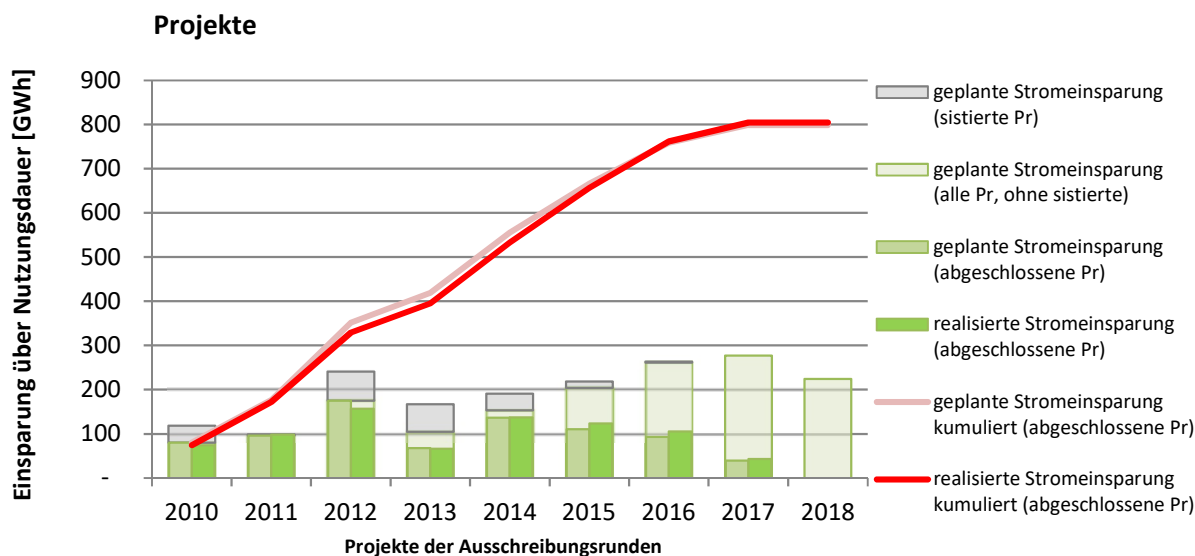
Abbildung 7: Erfolgskontrolle der Stromeinsparungen von Projekten
